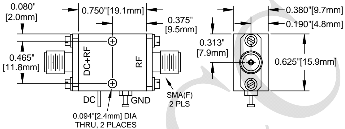
Fig. 2-A (Standard <> BT-XXXX-MS)
