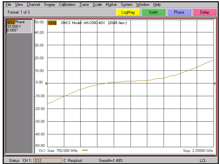
Phase Shift @ 20dB Attn.
