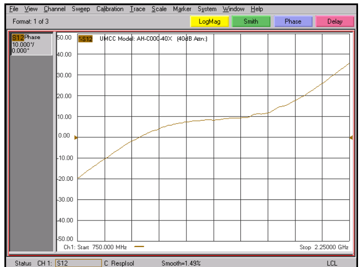
Phase Shift @ 40dB Attn.
