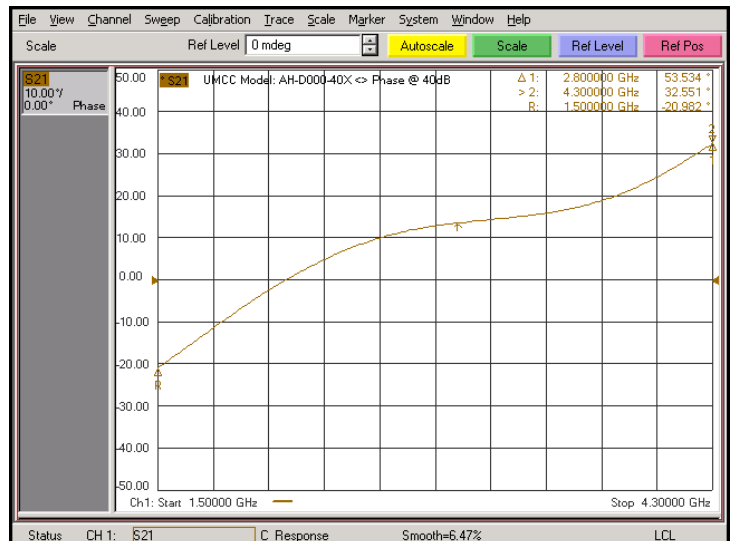
Phase Shift @ 40dB Attn.
