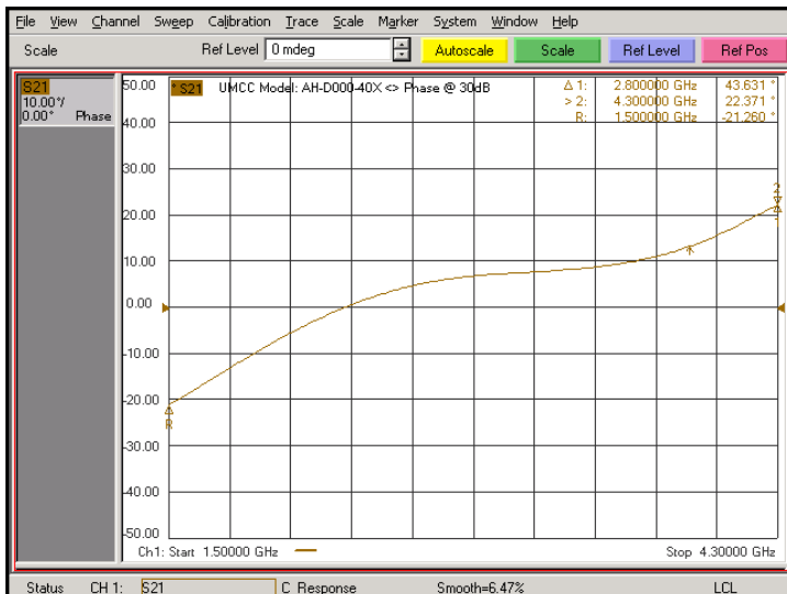
Phase Shift @ 30dB Attn.
