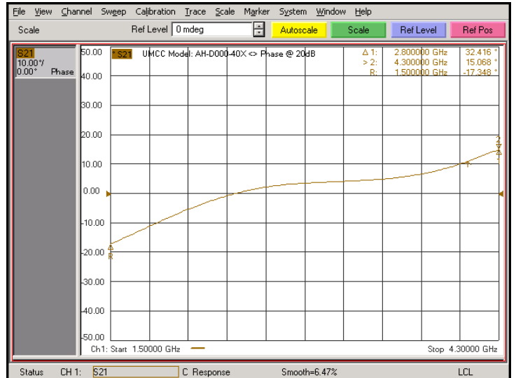
Phase Shift @ 20dB Attn.
