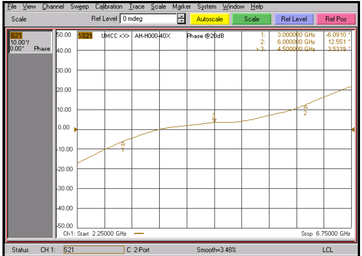
Phase Shift @ 20dB Attn.
