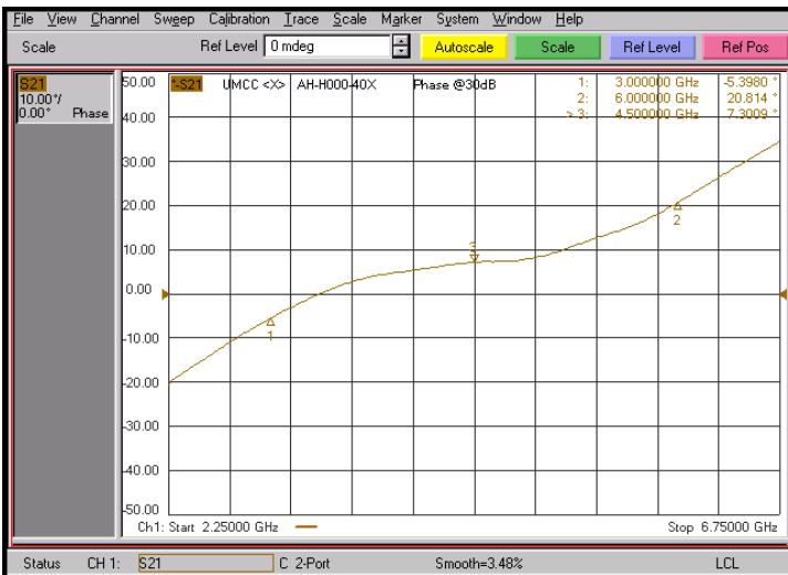
Phase Shift @ 30dB Attn.
