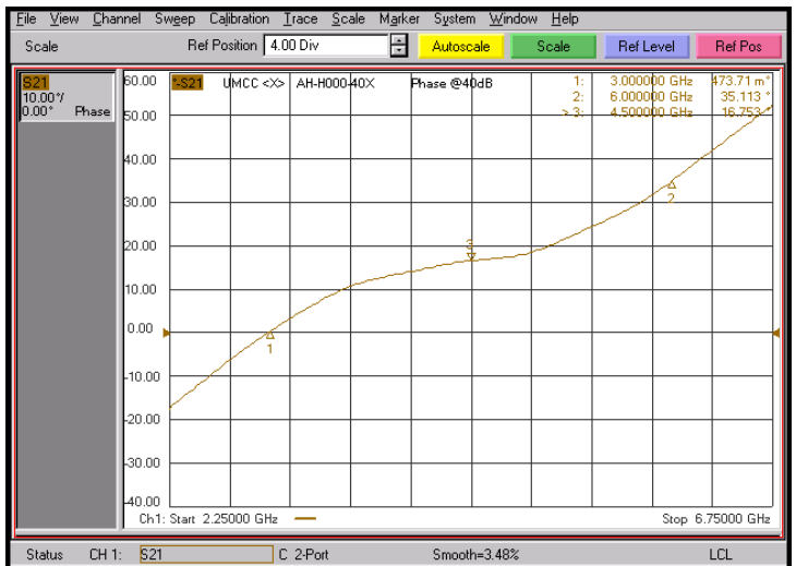
Phase Shift @ 40dB Attn.
