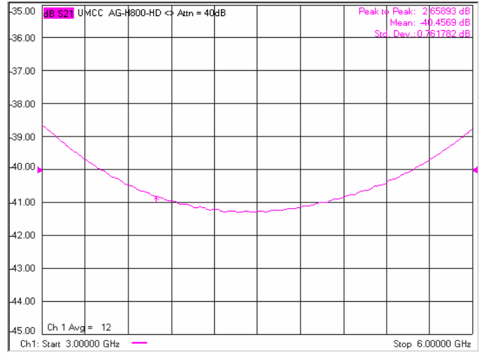
-Attenuation 40dB
