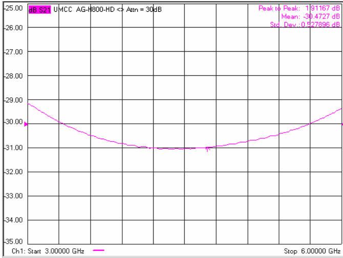
-Attenuation 30dB
