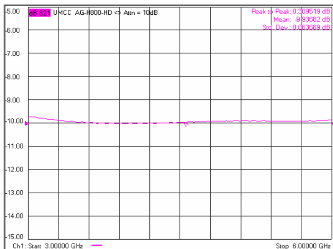
-Attenuation 10dB
