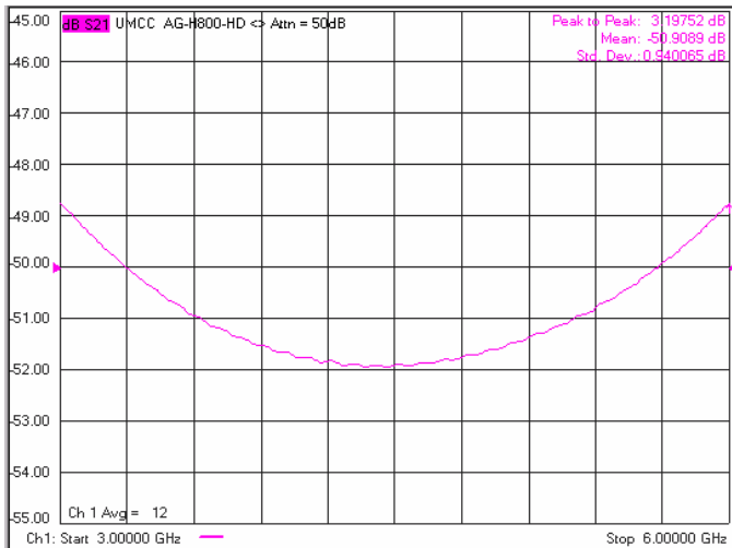
-Attenuation 50dB
