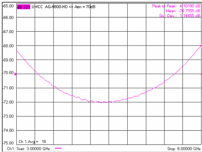
-Attenuation 70dB
