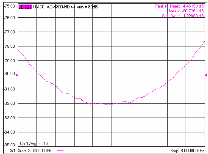
-Attenuation 80dB
