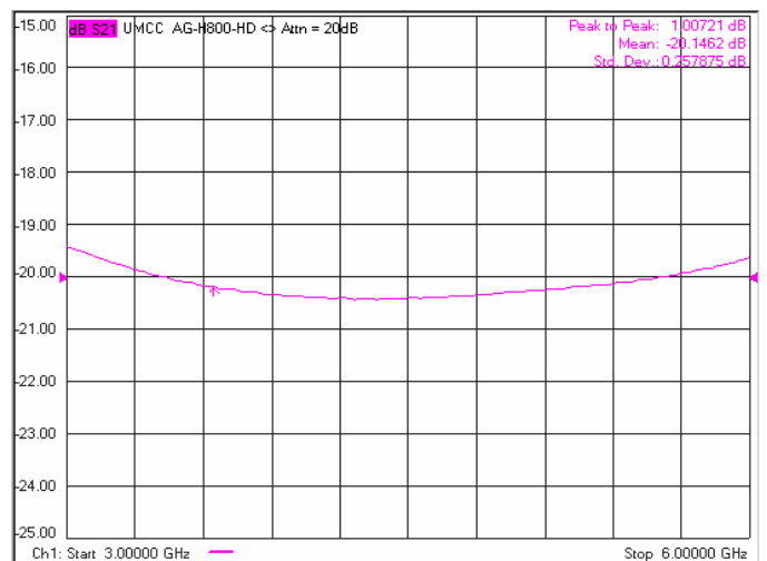
-Attenuation 20dB
