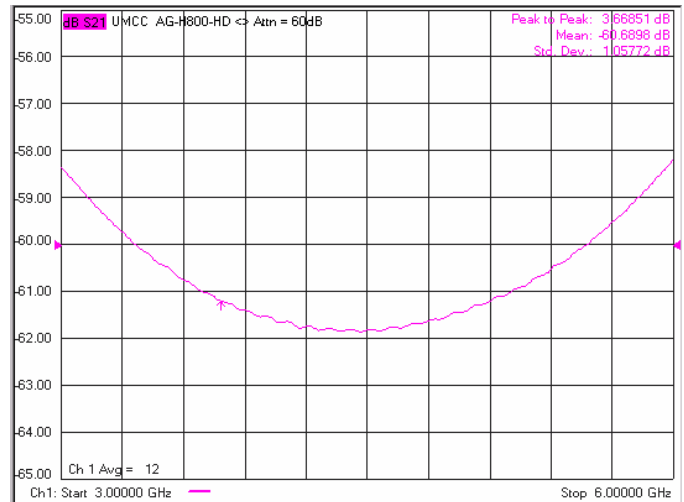
-Attenuation 60dB
