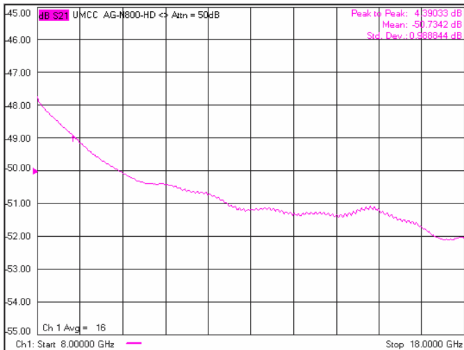
-Attenuation 50dB
