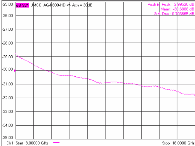
-Attenuation 30dB
