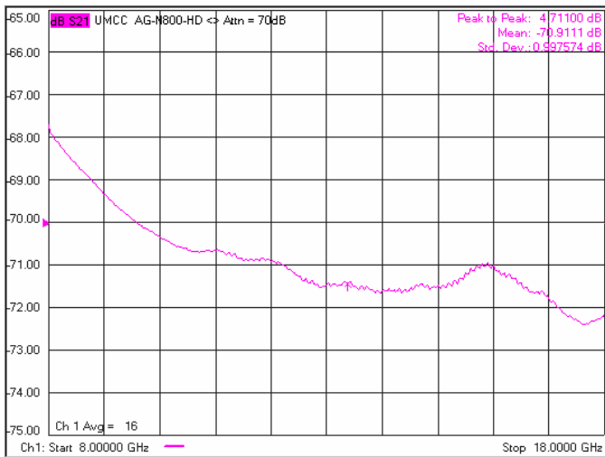
-Attenuation 70dB
