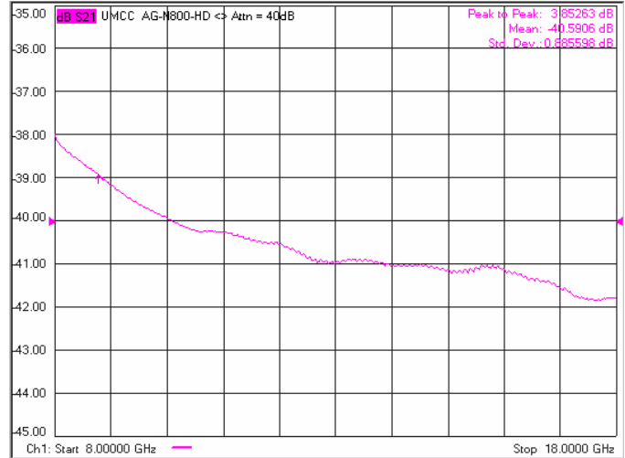
-Attenuation 40dB
