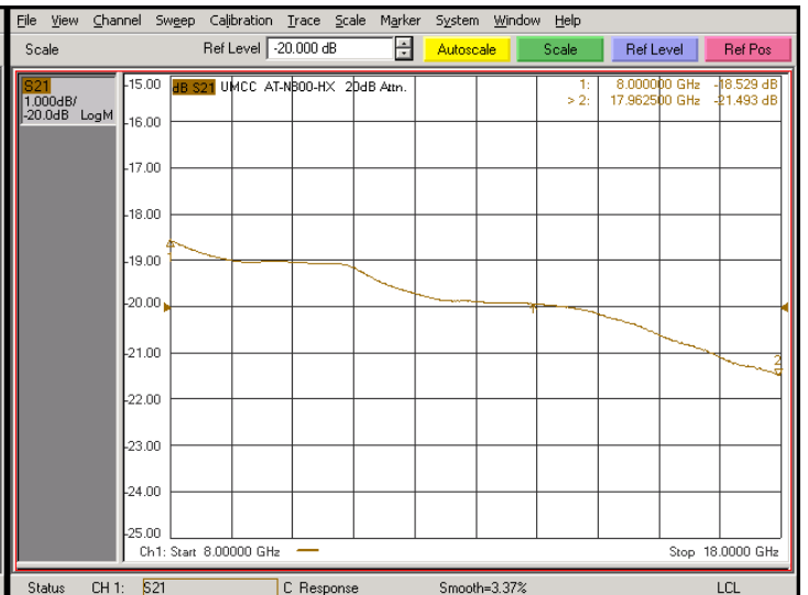
-Attenuation 20dB
