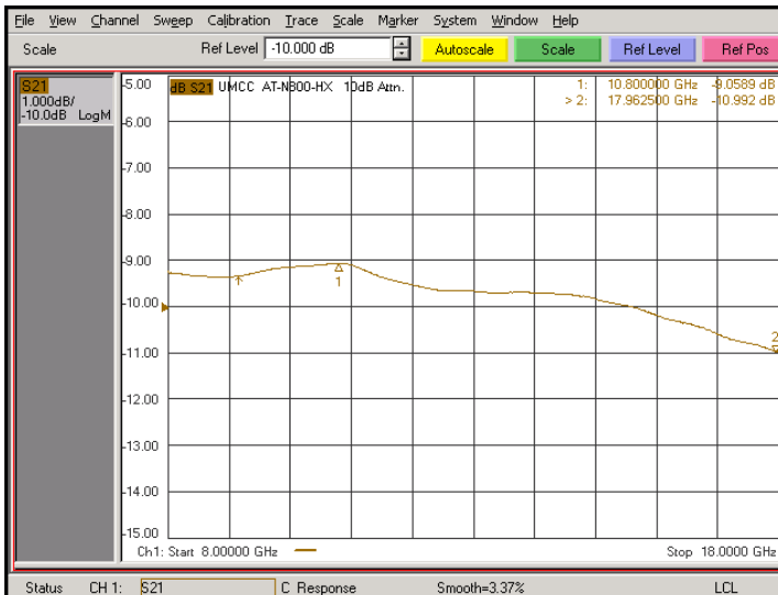
-Attenuation 10dB
